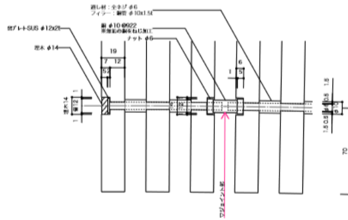
断面端部詳細図 1/2
