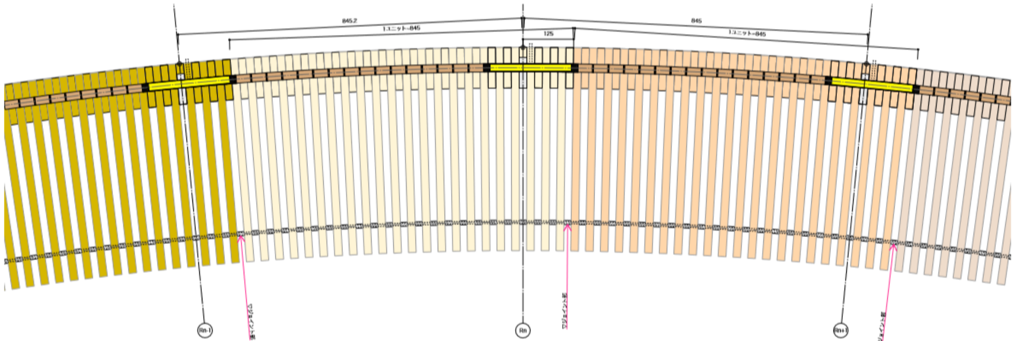
平面図
